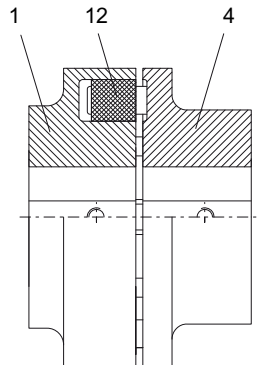
Figure 11-2 Dessin des pièces de rechange des types B et BDS
