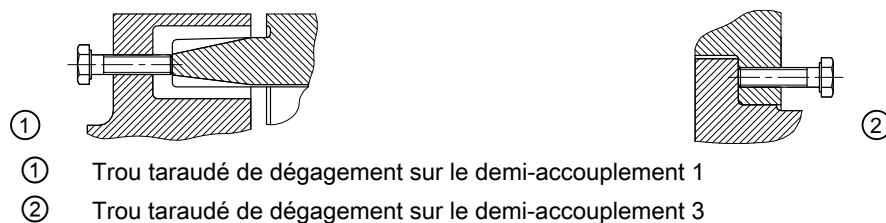
Figure 8-2 Trou taraudé de dégagement pour le desserrage du demi-accouplement 3 (3)
