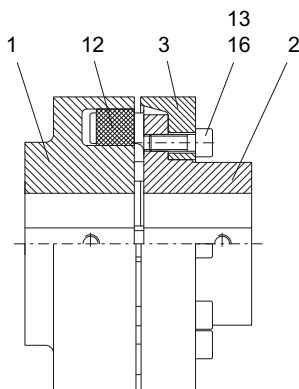
Figure 11-1 Dessin des pièces de rechange des types A et ADS
