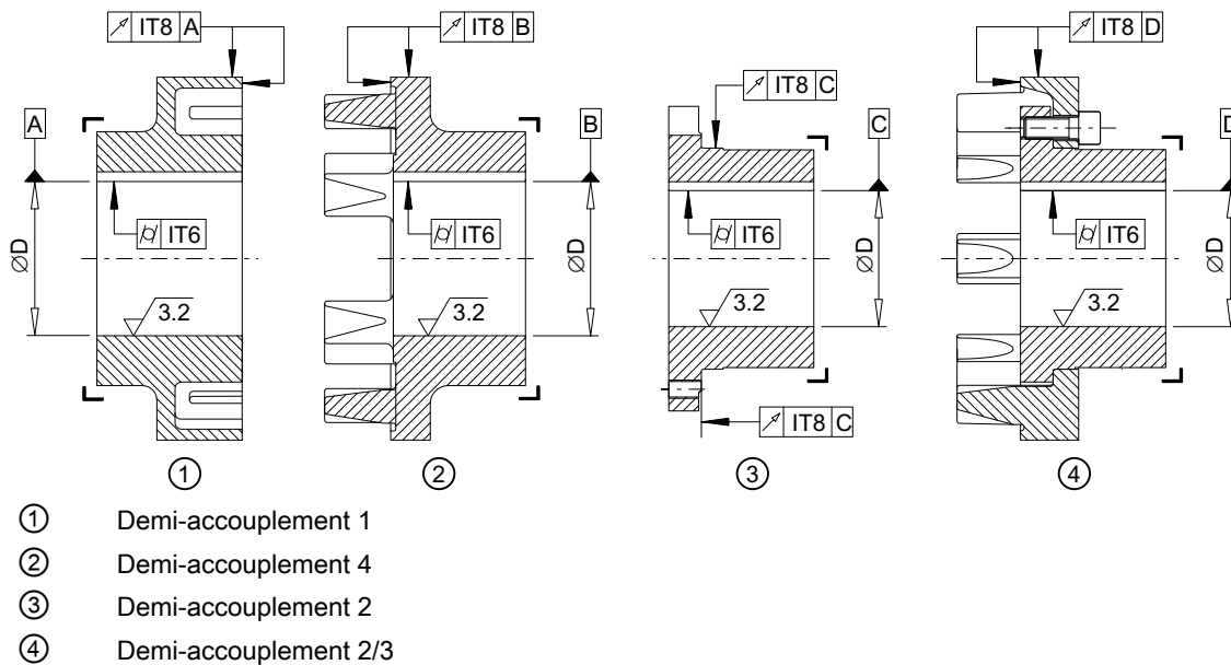
Figure 5-1 Tolérances de l'alésage fini
