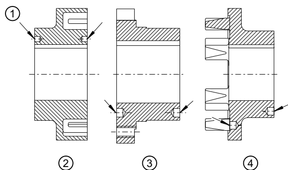
Figure 5-3 Position du trou d'équilibrage pour l'équilibrage à un plan
