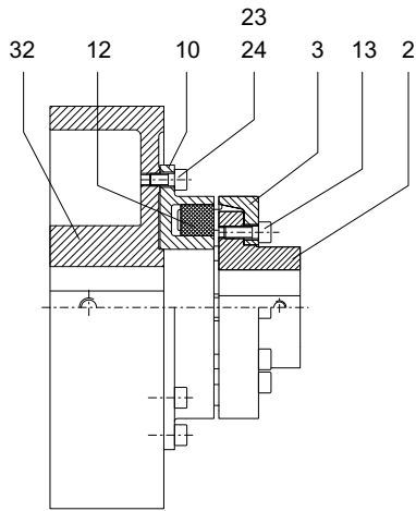
图 11-2 结构形式 P 的备件图纸
