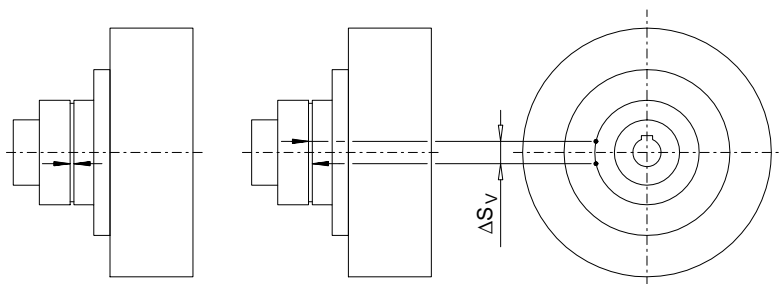
图 8-1 用于扭转间隙计算的标记
