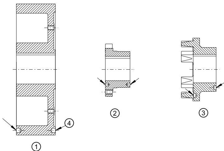
图 5-3 单平面平衡时平衡孔的位置
