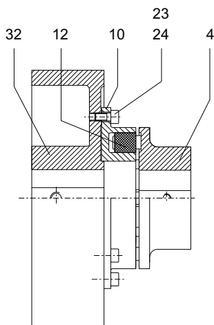
图 11-1 结构形式 O 的备件图纸
